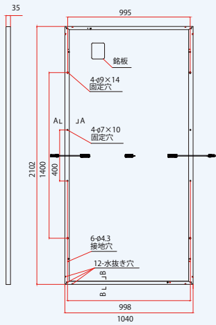
裏面図
